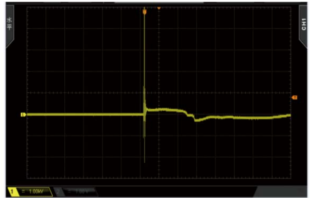
输出端电压波形 (共模 1.3KV)
