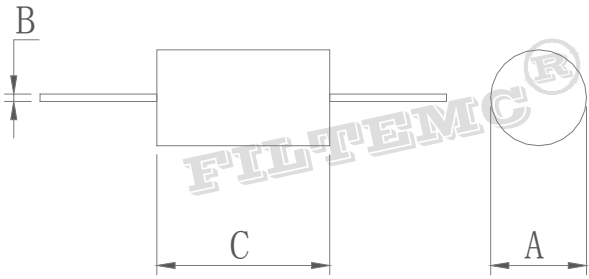
吸收磁珠 FT18/FT28
